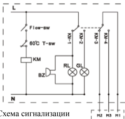
Выходы сигнализации
